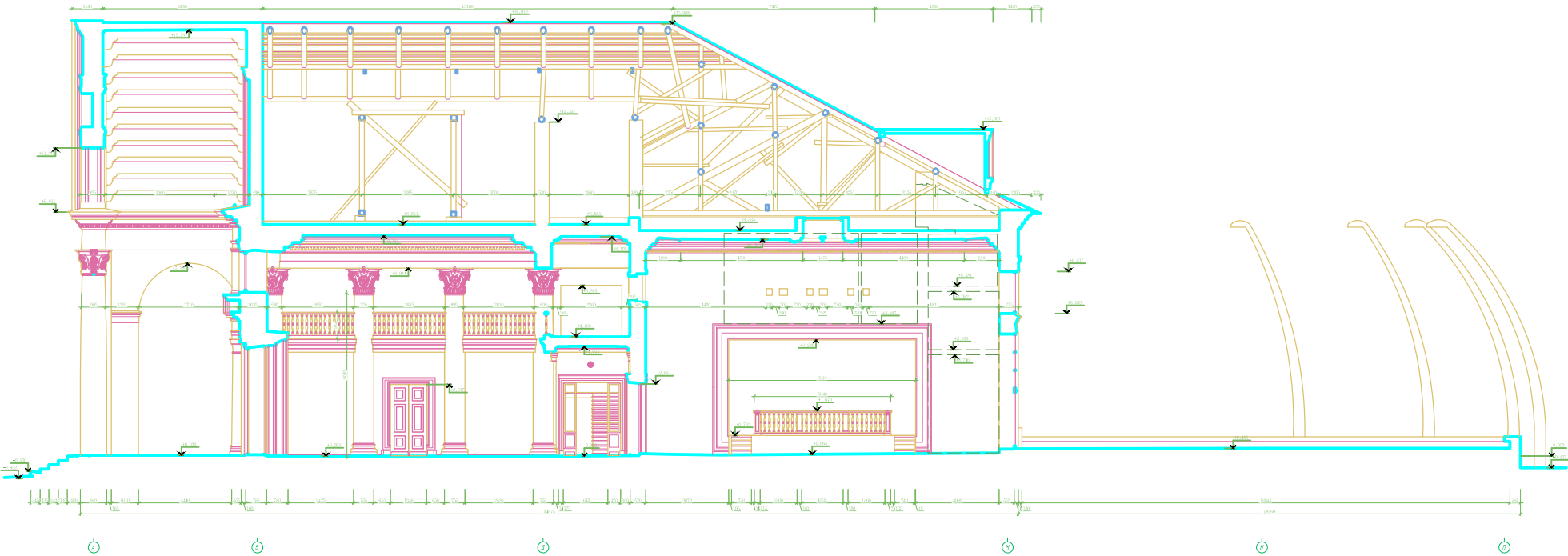
Разрез 1-1 в осях А-П М 1:50
